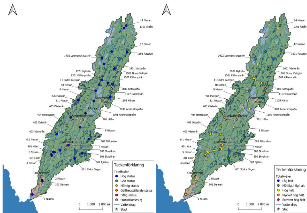
Figur 2. Status respektive tillstånd med avseende på medelhalten av totalfosfor och totalkväve (2020-2022) i Nissans avrinningsområde.
