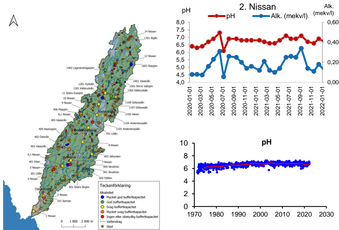
Figur 5. Vänster: Försumningstillstånd med avseende på buffertkapacitet (minimivärden 2020–2022). Stora prickar visar stationer provtagna av Nissans vattenråd samt punkt 1 provtagen inom den nationella miljöövervakningen. Små prickar visar provstationer från länens kalkeffektkontroll. Höger överst: pH och alkalinitet i provpunkt 2 vid Oskarström perioden 2020–2022. Nederst höger: pH-värden 1972–2022 i provpunkt Slottsmöllan. Den röda linjen visar glidande treårsmedelvärden.
