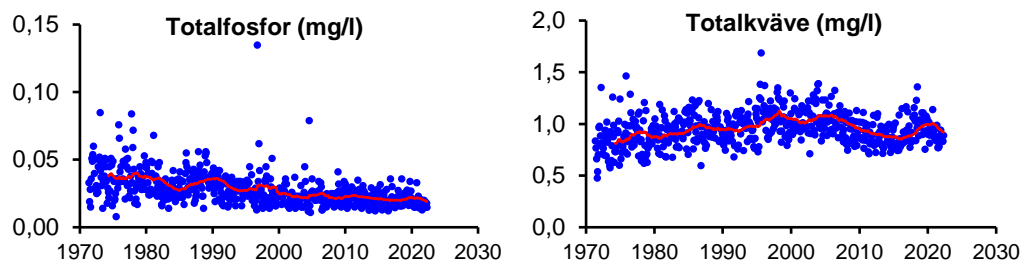
Figur 3. Halter av totalfosfor och totalkväve vid Slottsmöllan (nedersta provpunkten i Nissan) 1972 - 2022. Den röda linjen visar trenden som ett glidande treårsmedelvärde. Observera att axlarna är olika.
