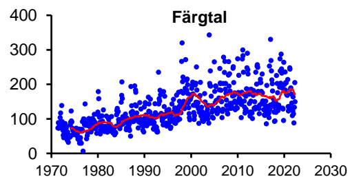
Figur 4. Vänster: tillståndet med avseende på vattnets färgtal i Nissans avrinningsområde (medelvärde 2020 – 2022). Överst höger: Medins utför sjöprovtagning. Nederst höger: Färgtalen vid Slottsmöllan (nedersta provpunkten i Nissan) 1972 - 2022.
