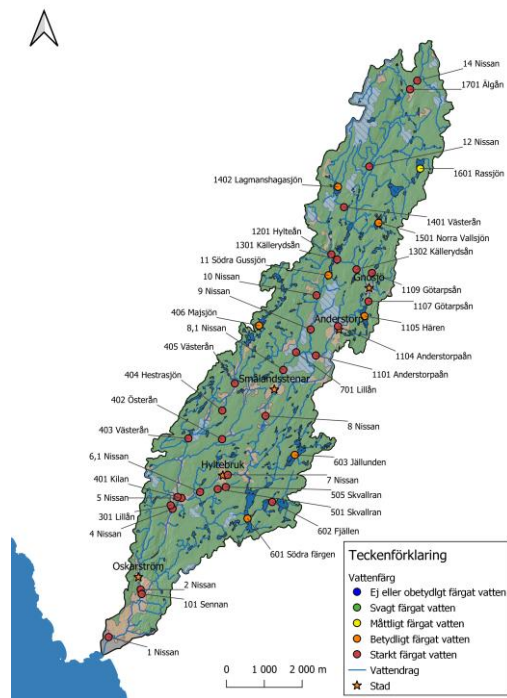
Figur 4. Vänster: tillståndet med avseende på vattnets färgtal i Nissans avrinningsområde (medelvärde 2020 – 2022). Överst höger: Medins utför sjöprovtagning. Nederst höger: Färgtalen vid Slottsmöllan (nedersta provpunkten i Nissan) 1972 - 2022.
